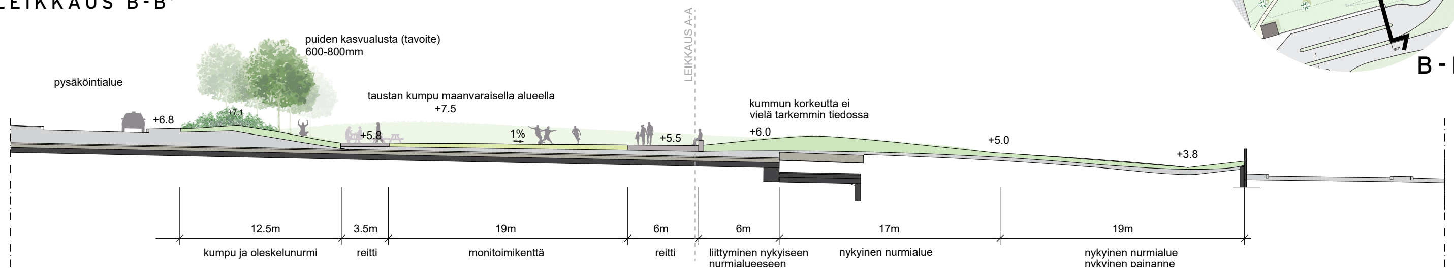
LEIKKAUS B-B'
